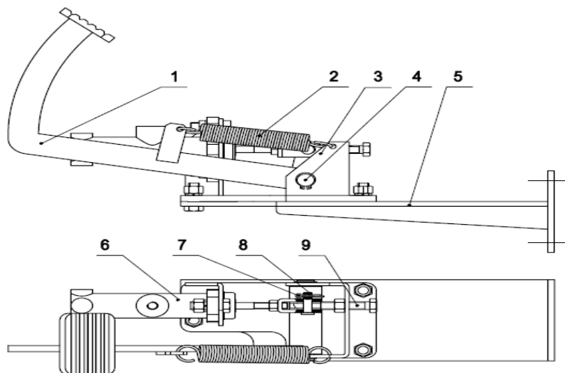
Рис. 10 – Ножной тормоз
